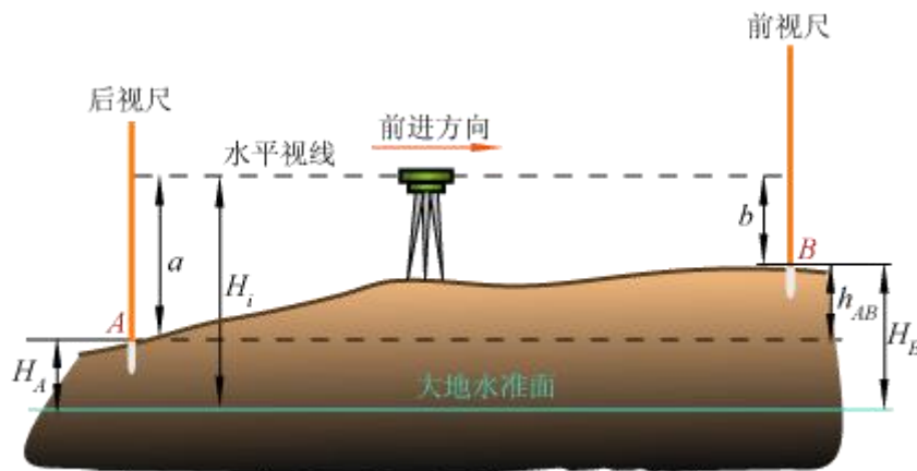
图2-1 水准测量原理
